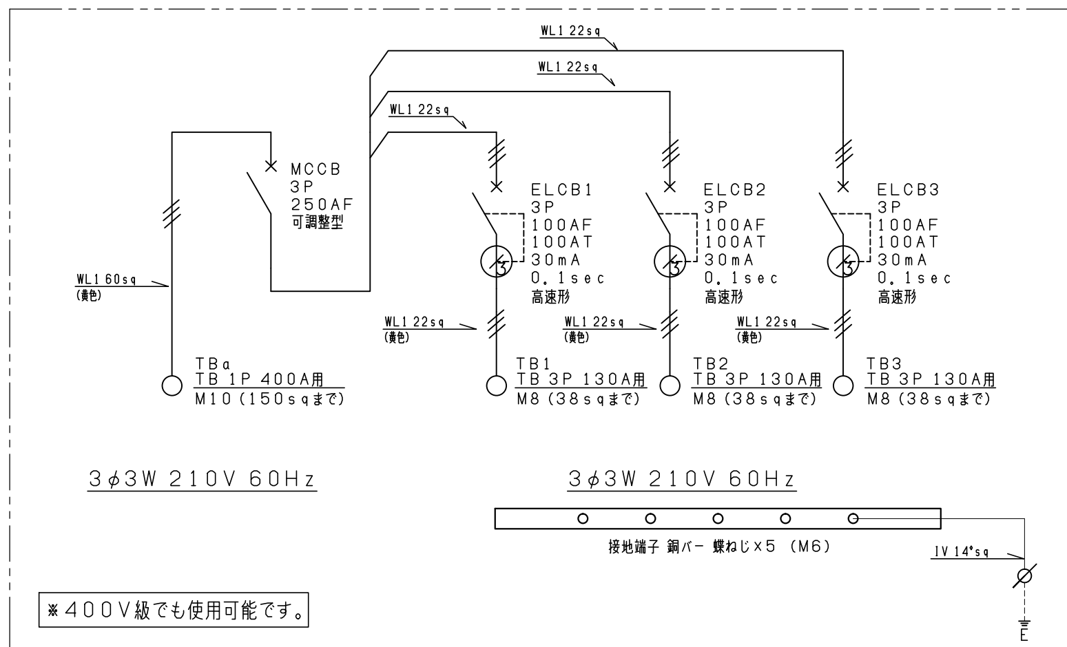
結線図
