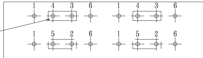
電圧切替片 (400V級使用時は 2枚重ねで使用)
