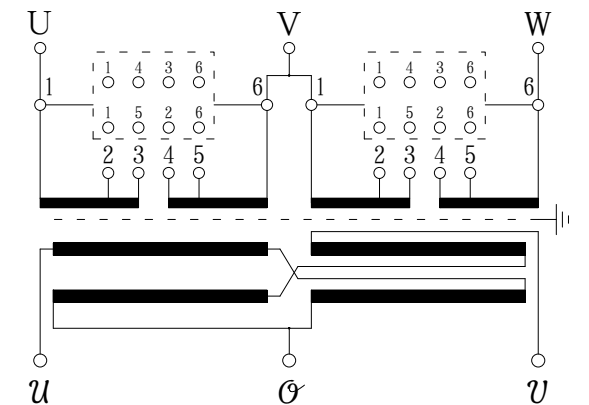
結線図
