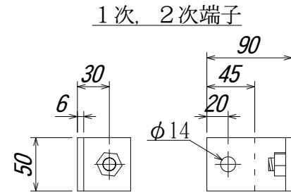
内部端子板詳細
